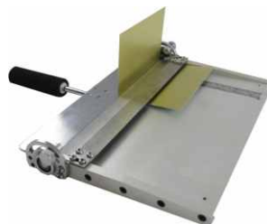
Plieuse à métal Pliage maximum Format A3 Largeur maximale des plaques : 30 cm Épaisseur des plaques : jusqu'à 1 mm Angles possibles : de 0 à 155°
